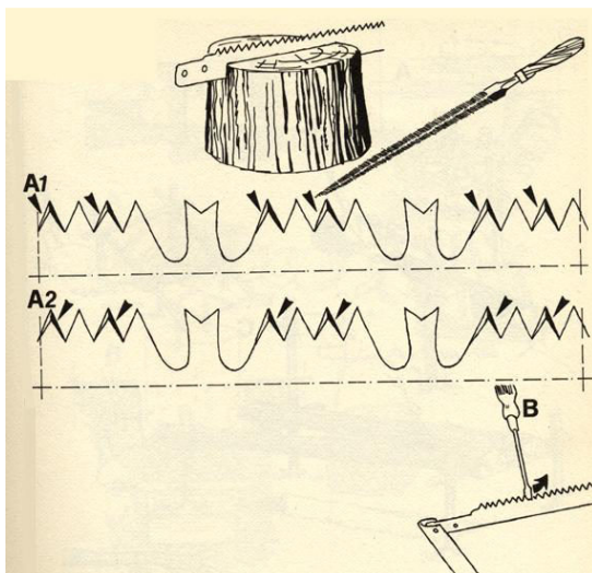
Schärfen eines Sägeblattes
